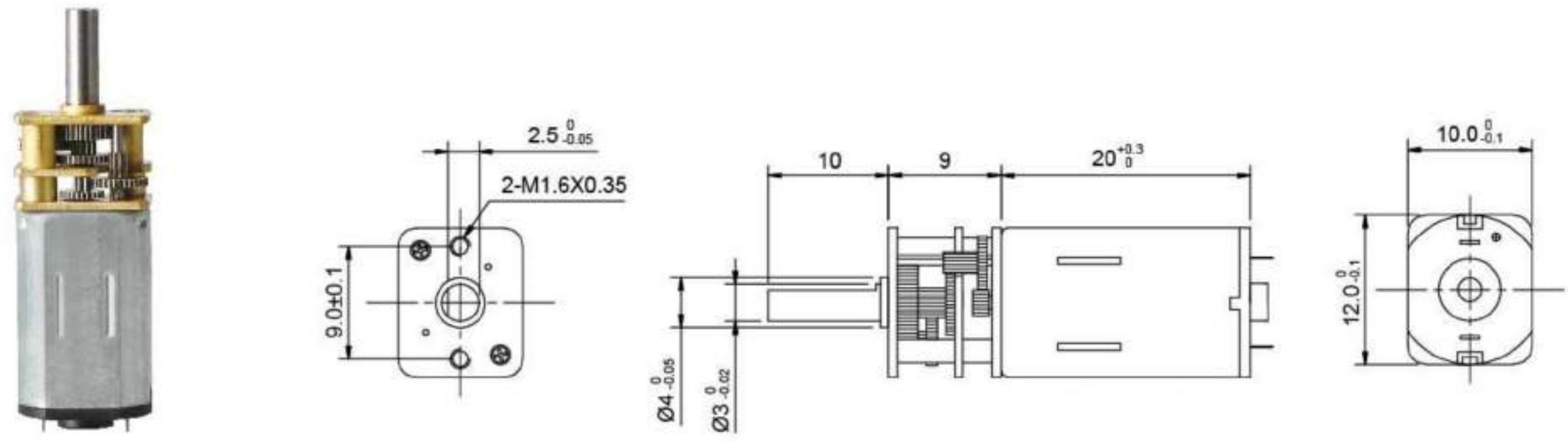
电机技术参数 Motor Technical Data
