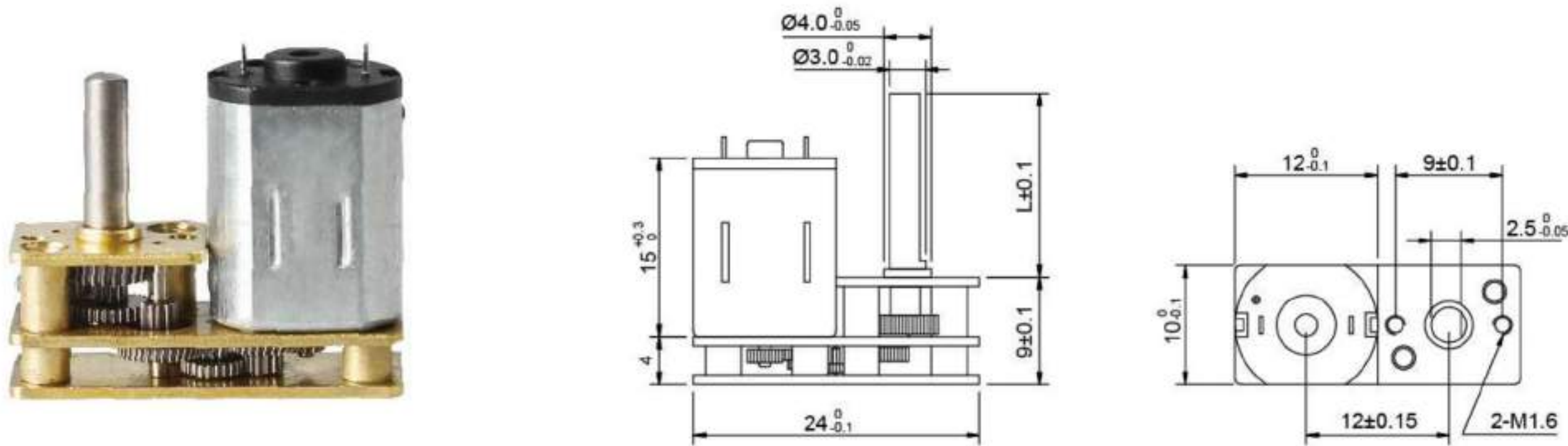
电机技术参数 Motor Technical Data
