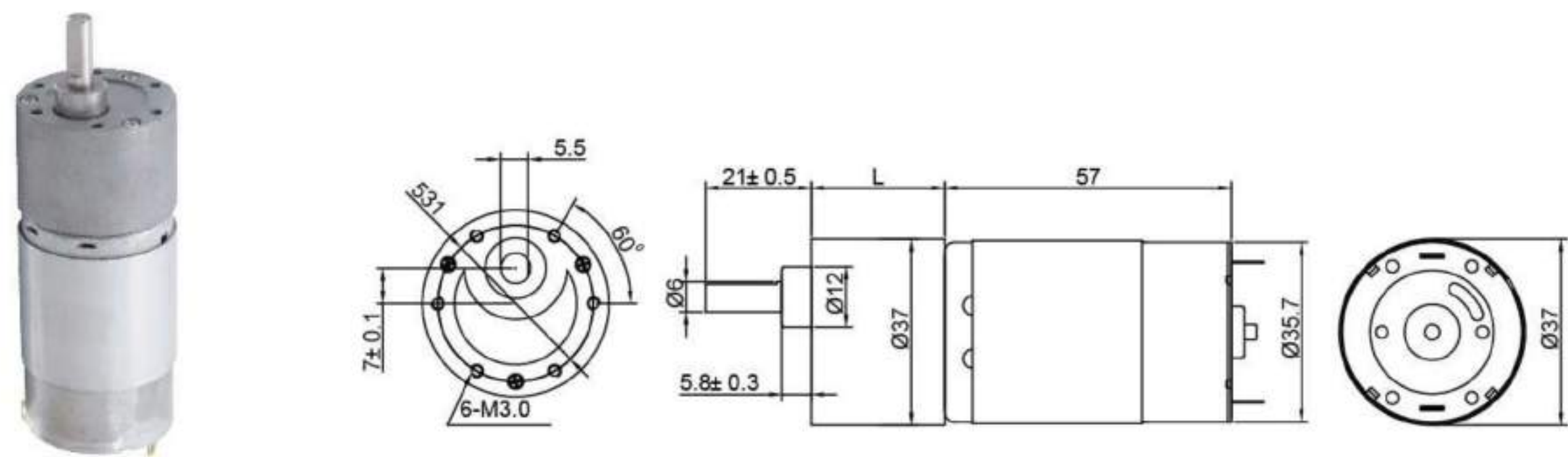
电机技术参数 Motor Technical Data
